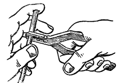
Рис. 22. Обжатие капсюля-детонатора на огнепроводном шнуре
