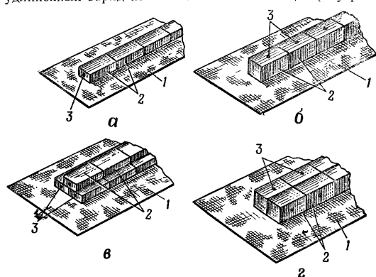
Рис. 14. Расположение тротильных шашек при изготовлении зарядов в тканевых оболочках: а — один ряд малых шашек; б — один ряд больших шашек; в — три ряда малых шашек; г — два ряда больших шашек; 1 — ткань; 2 — шашки; 3 — запальные гнезда
