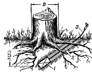
Рис. 75. Подрывание (выкорчевывание) пня: 1 — заряд; 2 — забивка; 3 — зажигательная трубка
