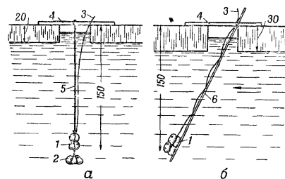
Рис. 241. Установка зарядов в прорубях при подрывании льда:
