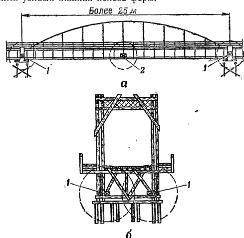
Рис. 135. Подрывание высоководного деревянного моста с гибкой аркой и балкой жесткости: а — вид сбоку; б — поперечный разрез; 1 — заряды над опорами; 2 — заряд в середине пролета
