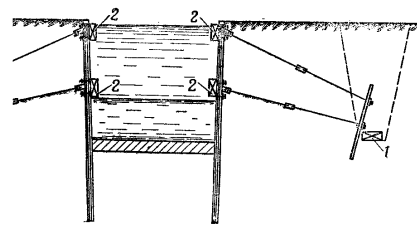
Подрывание шлюза с металлическими шпунтовыми стенками: 2 — заряды в колодцах у анкеров; 2 — заряды на шпунтовых стенах
