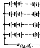
Рис. 61. Схема смешанного соединения элементов в батарею
