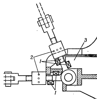
Подрывание гальсбантов шлюзовых ворот: 1 — заряд; 2 — гальсбанты; 3 — полотнище ворот
