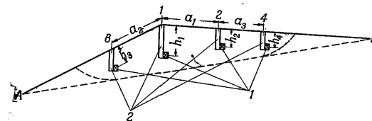
Рис. 102. Схема расположения зарядов для устройства съезда к переправе:
