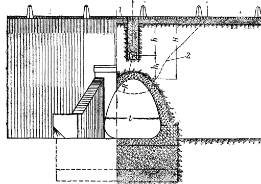
Рис. 190. Подрывание водопропускной трубы отверстием более 2,0 м 2 сосредоточенными зарядами в колодцах над сводами: 1 — заряд; 2 — контур ожидаемого рва
