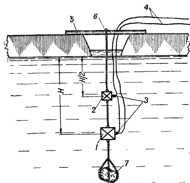
Рис. 242. Подрывание льда с применением забивочного заряда: 1 — основной заряд; 2 — забивочный заряд; 3 — электродетонаторы; 4 — провода; 5 — перекладина; 6 — веревка; 7 — груз
