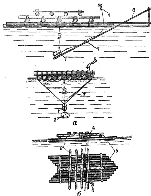
Рис. 139. Подорывание деревянных плотов: а — подводными сосредоточенными зарядами; б — надводными удлиненными зарядами; 1 — заряды; 2 — груз; 3 — шест; 4 — зажигательная трубка; 5 — поперечный; 6 — прогоны; 7 — детонирующий шнур
