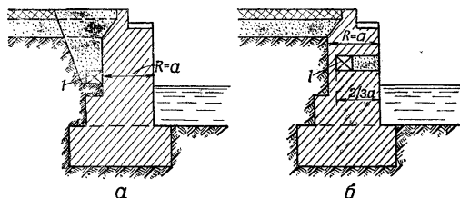
Рис. 152. Подрывание береговых мостовых опор (устоев) по всей ширине в одном уровне: а — сосредоточенными зарядами в колодцах; б — сосредоточенными зарядами в рукавах; I — заряды
