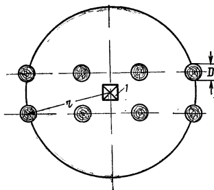
Рис. 74. Подрывание рассредоточенного куста свай неконтактным зарядом: 1 — заряд; r — радиус разрушения
