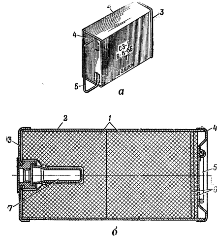
Рис. 3. Стандартный заряд СЗ-1:
