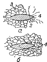
Рис. 246. Подрывание льда при постановке судна на плаву: а — положение судна до взрыва зарядов; б — то же, после взрыва зарядов; 1 — судно; 2 — заряды; 3 — битый лед; 4 — ледяное поле
