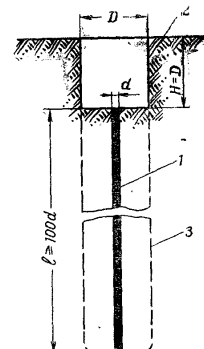
Рис. 115. Расположение удлиненного заряда в скважине с оголовком при устройстве шахтного колодца: 1 — заряд; 2 — оголовок скважины; 3 — расчетный контур колодца
