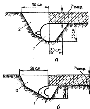
Рис. 185. Установкакумулятивных зарядов в приямки: а — заряд КЗ-2; б — заряд КЗУ; 1 — заряд; 2 — приямок
