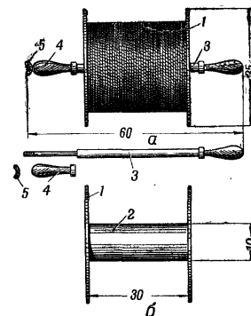
Рис. 271. Катушка для саперного провода КСП-2: а — в собранном виде с намотанным проводом; б — без провода в разобранном виде; 1 — щеки; 2 — барабан; 3 — ось; 4 — съемная ручка; 5 — барабек
