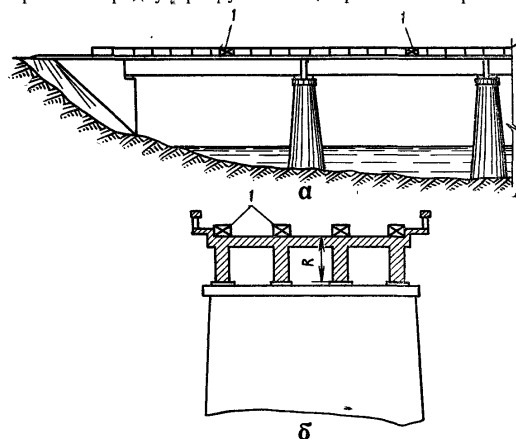
Рис. 160. Подрывание пролетных строений железобетонного балочного моста зарядами на проезжей части: а — вид сбоку; б — поперечный разрез; 1 — заряды
