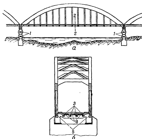
Рис. 164. Подрывание железобетонного моста с пролетным строением на безраспорных арках с затяжками;
