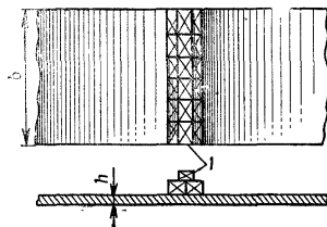
Рис. 76. Подрывание стального листа удлиненным зарядом: l — заряд из тротильных шашек; h — толщина листа; b — ширина листа
