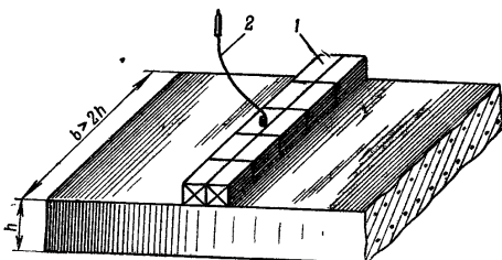
Рис. 90. Подрывание железобетонной плиты наружным удлиненным зарядом: 1 — заряд; 2 — зажигательная трубка
