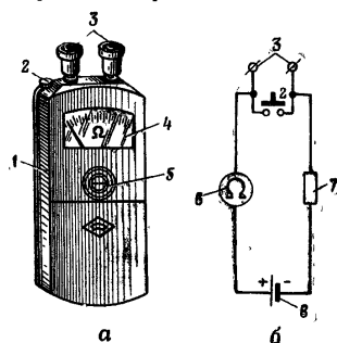
Рис. 49. Малый омметр М-57: а — общий вид; б — электрическая схема; 1 — корпус; 2 — кнопка для проверки омметра; 3 — клеммы; 4 — окошко со шкалой и стрелкой; 5 — головка корректора; 6 — индикатор; 7 — сопротивление; 8 — источник тока
