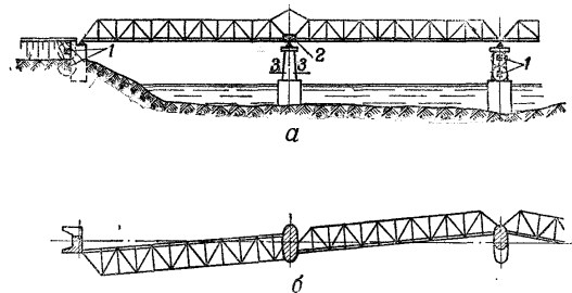
Рис. 145. Подрывание большепролетного металлического моста с пролетными строениями неразрезной конструкции: а — вид сбоку; б — план (после подрыва); 1 — заряды для подрывания концевых опор по косым сечениям; 2 — заряды для подрывания поясов ферм; 3-3 — сечения подрыва средних опор по всей ширине в одном уровне
