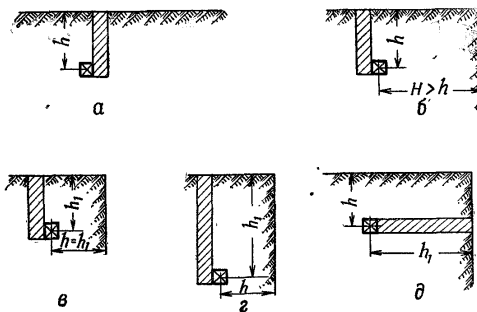
Рис. 94. Соотношения между линией наименьшего сопротивления h_1 и глубиной заложения заряда h :
