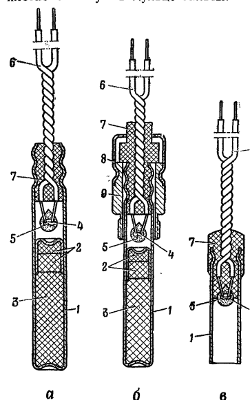
Рис. 34. Электродетонаторы: а — ЭДП; б — ЭДП-р; в — электровоспламенитель; 1 — гильза; 2 — заряд инициирующего ВВ; 3 — заряд ВВ повышенной мощности; 4 — платино-иридиевый мостик; 5 — воспламенительный состав; 6 — провода; 7 — пластиковая пробка; 8 — крышка; 9 — ниппель с резьбой
