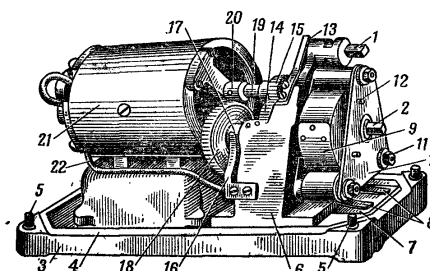
Рис. 44. Подрывная машинка ПМ-1 без кожуха:
