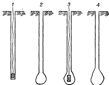
Рис. 104. Последовательность устройства зарядной камеры (котла) в шпуре: 1 — заряд для первого простреливания; 2 — результат первого простреливания; 3 — заряд для второго простреливания; 4 — результат второго простреливания
