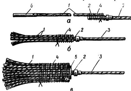
Рис. 27. Взрывание детонирующего шнура: а — взрывание одного конца шнура; б — взрывание от двух до шести концов шнура; в — взрывание от двух до шести концов шнура; 1 — концы детонирующего шнура; 2 — капсюль-детонатор зажигательной трубки; 3 — огнепроводный шнур; 4 — шпагат; 5 — шашка ВВ (буровая); 6 — капсюль-детонатор, вставляемый в заряд
