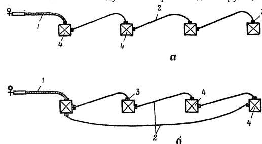
Рис. 30. Последовательная сеть детонирующего шнура: а — без замыкающего шнура; б — с замыкающим шнуром; 1 — зажигательные трубки; 2 — отрезки детонирующего шнура; 3 — капсули-детонаторы; 4 — заряды ВВ
