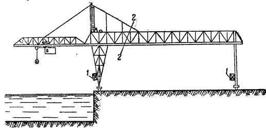
Рис. 226. Подрывание мостового крана: 1 — заряды на ногах крана; 2 — сечение подрыва фермы в пролете
