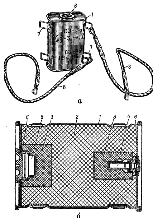
Рис. 5. Стандартный заряд СЗ-3а:
