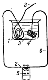
Рис. 36. Проверка изоляции саперного провода:
