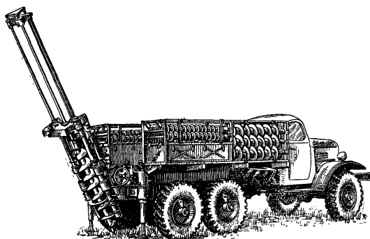
Рис. 273. Бурильная машина БГМ: а — при бурении вертикальной скважины; б — при бурении наклонной скважины
