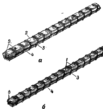
Рис. 11. Удлиненные заряды из тротильовых а — заряд в тканевой оболочке; б — заряд без обол; деревянных рейках; 1 — тротильовые шашки; 2 — тк- шпагат (мягкая проволока); 4 — деревянные рейки; ревяные колышки
