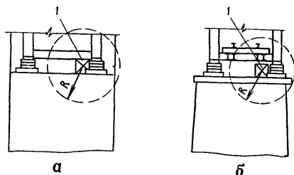
Рис. 155. Скалывание верхней части опор взрывом заряда на подферменной плите: а — расположение заряда на береговой опоре; б — расположение заряда на промежуточной опоре; 1 — заряд
