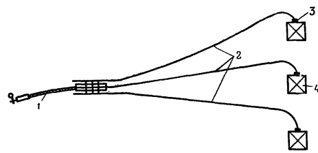
Рис. 31. Параллельная сеть детонирующего шнура: 1 — зажигательная трубка; 2 — отрезки детонирующего шнура; 3 — капсуль-детонатор; 4 — заряд ВВ
