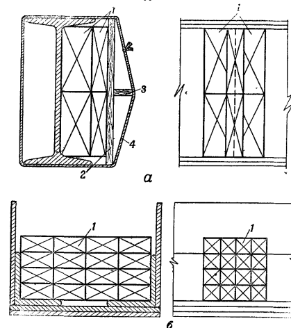
Рис. 79. Подрывание стальных балок сосредоточенными зарядами:
