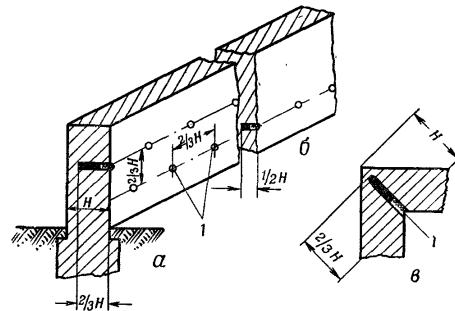
Рис. 119. Расположение шпуровых зарядов в стене:
