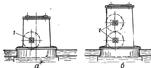
Рис. 154. Подрывание по косым сечениям мостовых опор малой ширины: а — при высоте опоры менее 15,0 м; б — при высоте опоры более 15,0 м; I — заряды
