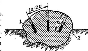
Рис. 109. Схема расположения шнуровых зарядов при дроблении крупного камня: 1 — заряды; 2 — забивка
