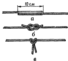
Рис. 29. Сروشки детонирующего шнура: а — внакладку; б — прямым узлом; в — двойной петлей
