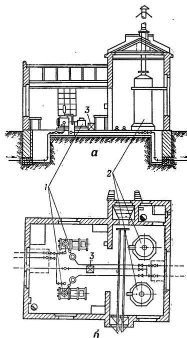
Рис. 205. Подрытие насосной станции: а — вертикальный разрез; б — план; 1 — насосы; 2 — паровые котлы; 3 — заряд
