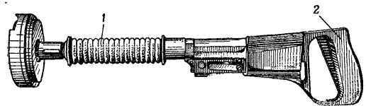
Рис. 279. Строительно-монтажный пистолет СМП-3: 1 — ствол; 2 — рукоятка
