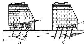
Рис. 151. Забивка зарядов в быках: а — сосредоточенных зарядов в нишах; б — удлиненного заряда в борозде; 1 — щиты из досок; 2 — доски; 3 — подпорки
