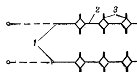
Рис. 55. Схема электровзрывной сети с последовательным соединением групп, состоящих из попарно-параллельно соединенных электродетонаторов: 1 — магистральные провода; 2 — участковые провода; 3 — электродетонаторы
