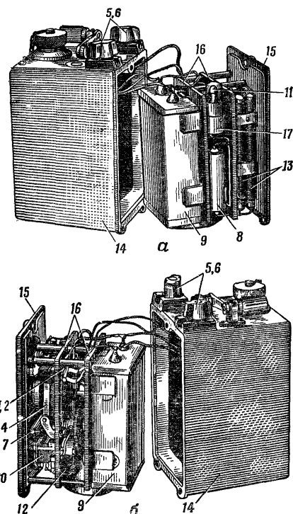
Рис. 38. Конденсаторная подрывная машинка КРМ-1, вынутая из корпуса:
