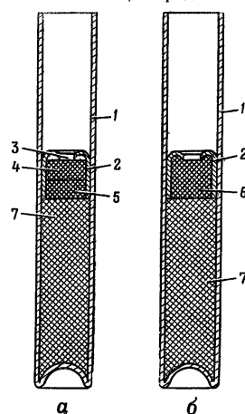
Рис. 18. Капсюли-детонаторы: а — № 8-А; б — № 8-М; 1 — гильза; 2 — чашечка; 3 — сетка; 4 — тенерес; 5 — азид свинца; 6 — ртуть; 7 — тетрил (тэн или гексоген)
