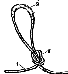
Рис. 63. Предохранительная петля на участке сростка саперного провода: 1 — провод; 2 — сросток; 3 — узел
