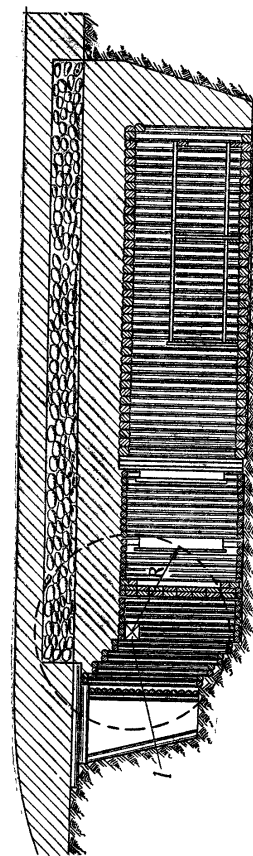
Рис. 229. Подрывание убежища тяжелого типа I — заряд; R — расчетный радиус разрушения
