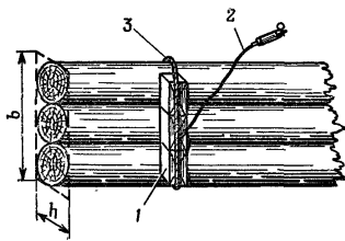
Рис. 72. Подрывание плоского пакета бревен наружным зарядом:
