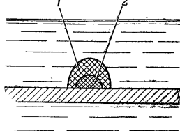
Рис. 87. Перебивание стального листа под водой кумулятивным удлиненным зарядом с защищенной полостью: 1 — заряд; 2 — вкладыш из пенопласта
