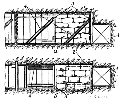
Рис. 113. Устройство забивки в галерее: а — продольный разрез; б — план; 1 — заряд; 2 — мешки с грунтом; 3 — щиты из досок; 4 — подпорки
