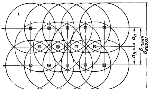
Рис. 101. Схема расположения сосредоточенных зарядов в три ряда
