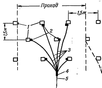
Рис. 233. Устройство прохода в надолбах: 1 — надолбы; 2 — заряды; 3 — детонирующий шнур; 4 — шашка ВВ; 5 — зажигательная трубка
