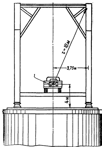
Рис. 264. Схема расположения резервного заряда на подрываемом металлическом мосту; I — заряд в кузове автомобиля
