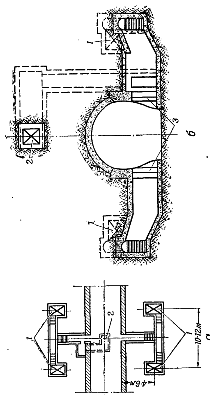
Рис. 178. Боковые галереи с зарядными камерами, устраиваемые в туннелях, проходящих в твердых породах: а — план; б — поперечный разрез; 1 — боковые зарядные камеры; 2 — верхняя зарядная камера; 3 — двери, закрывающие входы в галереи
