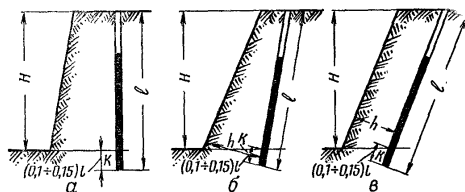
Рис. 111. Типы зарядных скважин: а — вертикальная скважина; б — скважина под углом к откосу уступа; в — скважина, параллельная откосу уступа; к — перебур
