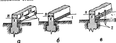
Рис. 116. Подрывание бескаркасных стен наружными зарядами:
