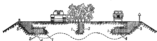
Рис. 183. Закладка зарядов для подрывания земляного полотна дороги в горизонтальные галереи: 1 — заряды; 2 — контуры ожидаемых воронок; 3 — забивка; 4 — крепление галерей
