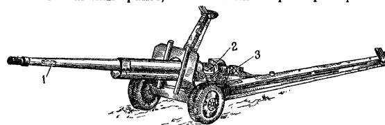
Рис. 237. Подрывание артиллерийского орудия: 1 — заряд в канале ствола; 2 — заряд в патроннике; 3 — заряд у затвора
