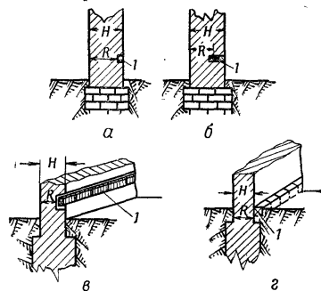
Рис. 117. Подрывание бескаркасных стен внутренними зарядами:
