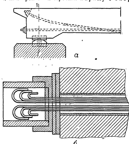
Рис. 161. Подрывание предварительно напряженной железобетонной балки:
