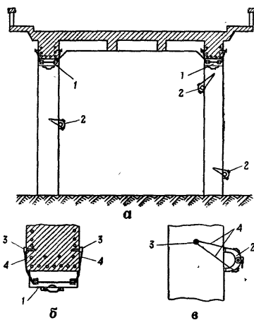
Рис. 167. Подрывание железобетонного путепровода удлиненными кумулятивными зарядами КЗУ: а — расположение зарядов на стойках и балках; б — крепление заряда на балке; в — крепление заряда на стойке; 1 — заряды; 2 — штыри (дюбели), забитые выстрелами из строительного пистолета; 3 — проволока
