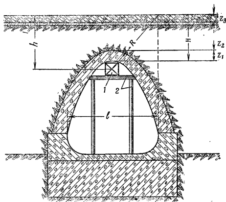
Рис. 191. Подрывание водопропускной трубы отаерствием более 2,0 м 2 зарядами, расположенными под сводом: 1 — заряд; 2 — подмости для заряда
