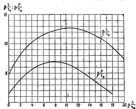
Рис. 96. График для определения размеров воронок при взрыве ядерных зарядов в грунте
