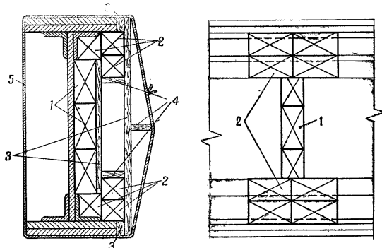
Рис. 88. Подрывание двутавровой балки фигурным зарядом под водой:
