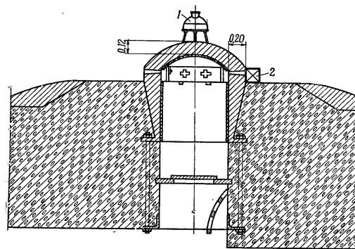
Рис. 228. Пробивание броневых закрытий фортификационного сооружения:
