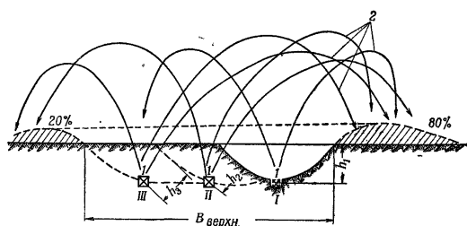
Рис. 106. Схема расположения зарядов для направленного выброса грунта (при разновременном взрывании): I — заряды; 2 — направление выброса основной массы грунта; I, II, III — последовательность взрывания зарядов
