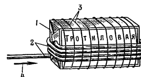
Рис. 28. Тротиловая шашка, подготовленная к бескапсюльному взрыванию детонирующим шнуром «боевик»: 1 — тротиловая шашка; 2 — детонирующий шнур; 3 — шпагат; 4 — направление детонации
