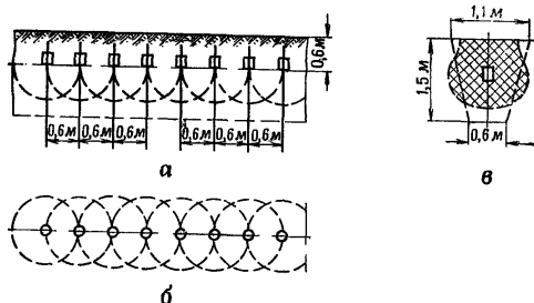
Рис. 257. Схема расположения зарядов для рыхления мерзлого грунта при устройстве траншей: а — продольный разрез; б — план; в — поперечный разрез
