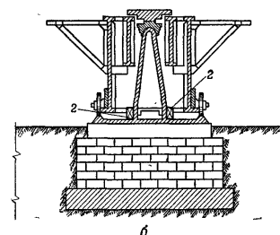
Рис. 209. Подрывание поворотного круга: а — вертикальный разрез; б — детали поворотной оси; 1 — заряды у катков; 2 — заряды у поворотной оси; 3 — заряд на ферме
