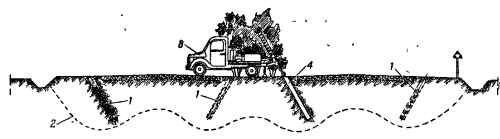
Рис. 184. Закладка зарядов для подрывания земляного полотна дороги в наклонные скважины: 1 — заряды; 2 — контур ожидаемого рва; 3 — бурильная машина; 4 — скважина
