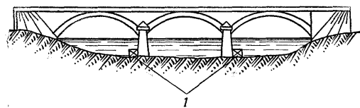
Рис. 166. Подрывание низких опор арок железобетонных мостов подводными зарядами;
