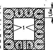
Рис. 126. Обрушение башни на месте путем подрывания всех стен шпуровыми зарядами: I — заряды
