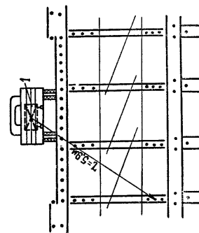
Рис. 261. Схема расположения резервного заряда на подрываемом деревянном мосту: 1 — заряд на волокуше в кузове автомобиля
