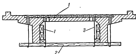
Рис. 168. Крепление наружных зарядов на конструкциях железобетонного моста: 1 — заряды; 2 — доска; 3 — жгуты из проволоки
