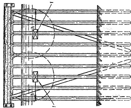
Рис. 224. Подрывание железобетонного пирса: 1 — заряд
