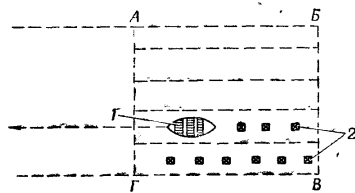
Рис. 247. Установка зарядов на дно реки с лодки: 1 — лодка; 2 — заряды; АБВГ — участок подрывных работ
