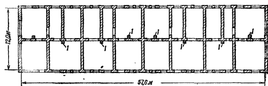
Рис. 125. Обрушение здания на месте взрывом неконтактных зарядов, расположенных на полу первого этажа: I — заряды
