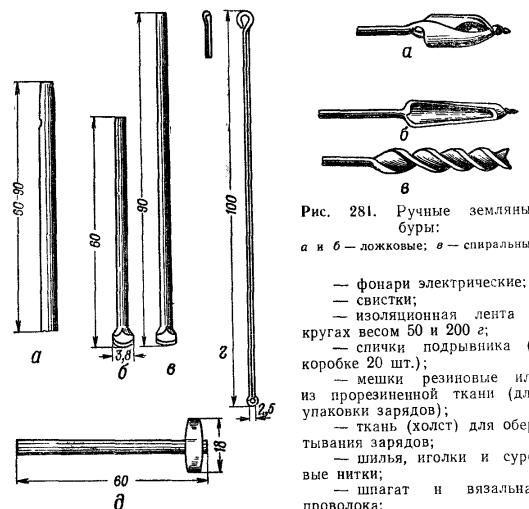
Рис. 280. Инструменты для ручного бурения: a — шлямбур; б и в — сверла; г — ложка для прочистки шпуров; д — молоток
