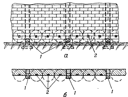
Рис. 121. Подрывание каркасной стены сосредоточенными зарядами:
