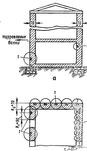
Рис. 124. Валка здания в сторону путем подрывания стен: а — поперечный разрез здания; б — план; I — заряды
