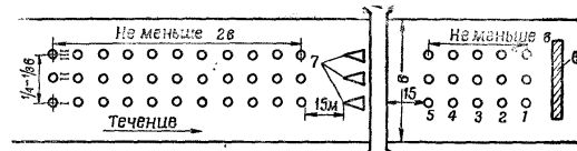
Рис. 244. Расположение лунок для зарядов при устройстве канала во льду:
