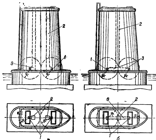
Рис. 156. Расположение зарядных камер в колодцах, устраиваемых в опорах мостов: а — при двух колодцах в опоре; б — при одном колодце; 1 — зарядные камеры; 2 — колодцы; 3 — рукава
