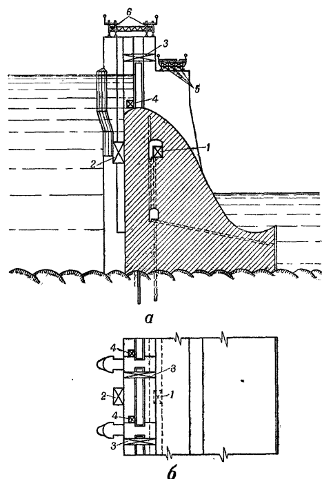
Рис. 212. Подрывание бетонной плотины с массивным водосливом:
