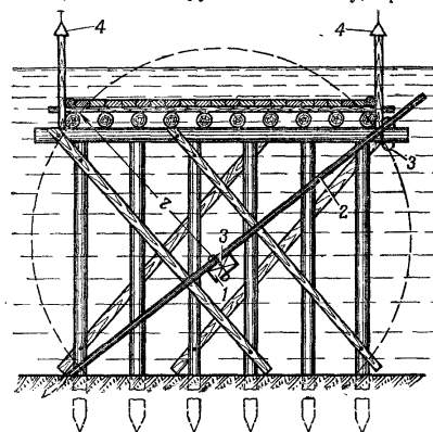
Рис. 173. Подрывание подводного деревянного моста подводными зарядами: 1 — заряд; 2 — шест; 3 — вязальная проволока или веревка; 4 — указки (вехи)
