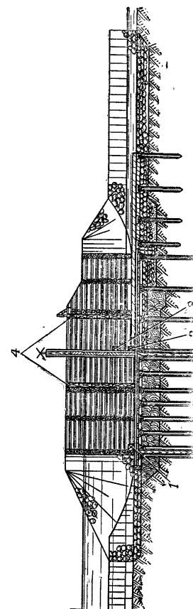
Рис. 218. Подрывание деревянной плотины (водослива): 1 — заряд у опорного узла; 2 — заряд у коронного узла; 3 — заряд у опорной стойки шпала; 4 — заряды на стенке сруба
