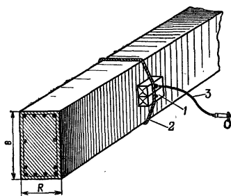
Рис. 89. Подрывание железобетонной балки наружным сосредоточенным зарядом: 1 — заряд; 2 — веревка (провока); 3 — зажигающая трубка
