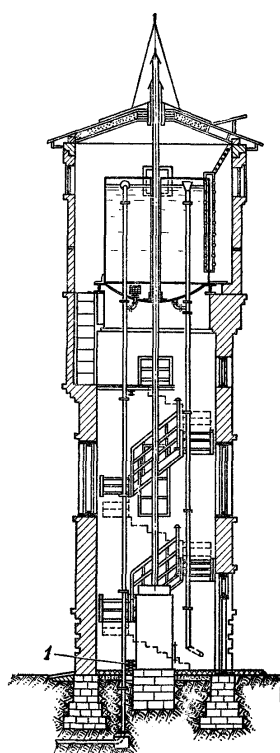
Рис. 206. Подрывание водонапорной башни: 1 — заряд
