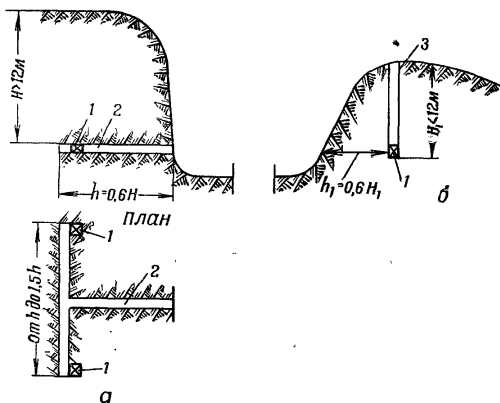
Рис. 112. Схема расположения камерных зарядов: а — в галерее; б — в колодце; 1 — заряд; 2 — галерея; 3 — колодец
