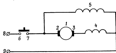
Рис. 45. Электрическая схема подрывной машинки ПМ-1:
