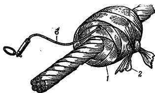
Рис. 85. Подрывание стального троса кольцевым зарядом из пластичного ВВ: 1 — заряд из пластика; 2 — крепление заряда бинтом или тканевой лентой; 3 — зажигающая трубка
