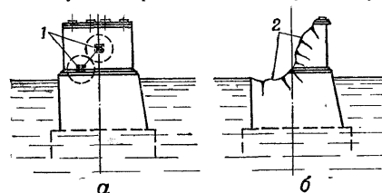
Рис. 153. Подрывание мостовой опоры по косому сечению с целью сбрасывания пролетного строения: а — расположение зарядов; б — подорванная опора; I — заряды; 2 — линия обрушения
