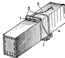
Рис. 92. Расчлененное расположение заряда на подрываемой железобетонной балке:
