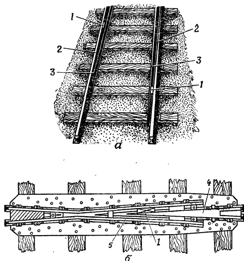
Рис. 199. Подрывание стрелочного перевода: а — стрелка; б — крестовина; 1 — заряды; 2 — рамные рельсы; 3 — остряки; 4 — сердечник; 5 — усовик
