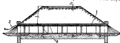
Рис. 189. Подрывание удлиненным зарядом водопропускной трубы отверстием до 2,0 м 2 :
