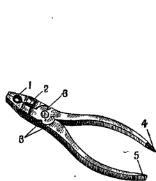
Рис. 269. Комбинированный обжим:
