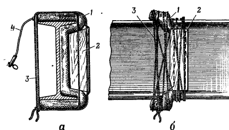
Рис. 78. Подрывание стальной балки зарядом из пластичного ВВ:
