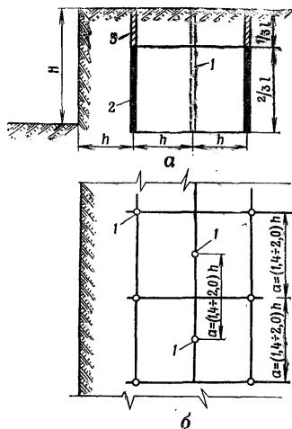
Рис. 108. Схема расположения шпуровых зарядов в массиве разрабатываемой породы: а — вертикальный разрез; б — план; 1 — шпуры; 2 — заряды; 3 — забивка
