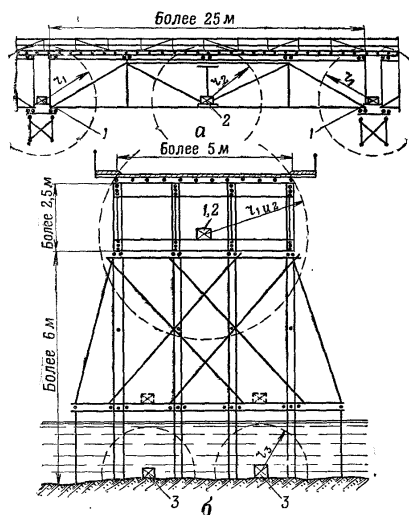
Рис. 133. Подрывание высоководного деревянного моста с ригельно-раскосными фермами: а — вид сбоку; б — поперечный разрез; 1 — заряды над опорами; 2 — заряд в середине пролета; 3 — заряды под водой (пунктиром показано положение зарядов до погружения в воду)
