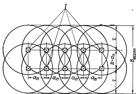
Рис. 100. Схема расположения сосредоточенных зарядов в два ряда: 1 — заряды
