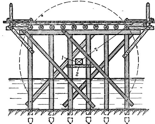
Рис. 130. Подрывание опор и пролетных строений низководных деревянных мостов: 1 — заряд; 2 — подмости для укладки заряда
