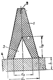
Рис. 17. Сосредоточенныйкумулятивный заряд из пластита-4: 1 — заряд ВВ; 2 — запальное гнездо; 3 —кумулятивная полость; 4 —пробиваемая плита
