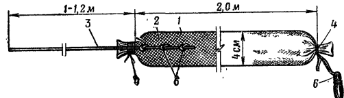
Рис. 15. Удлиненный заряд из пластина-4 с отрезком ДШ: 1 — оболочка из ткани; 2 — пластина-4; 3 — отрезок ДШ; 4 — завязка шпигатом; 5 — узлы на ДШ; 6 — конец шпигата для связывания зарядов
