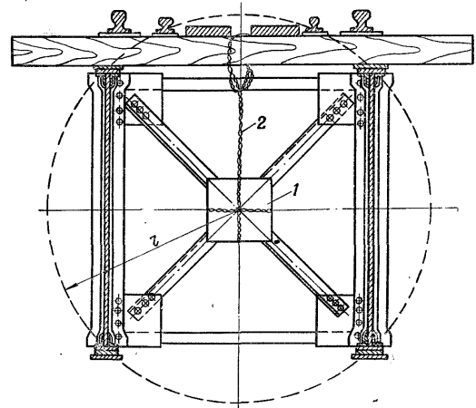
Рис. 143. Подрывание неконтактными зарядами металлических пролетных строений со сплошными фермами: 1 — заряд; 2 — проволоочная или веревочная подвеска
