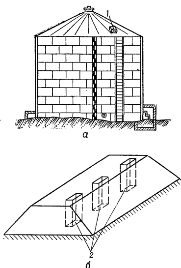
Рис. 210. Уничтожение пристанционных складов горячего: а — подрывание бензохранилища; б — сжигание угольного штабеля; 1 — заряд на крыше резервуара; 2 — колодцы в штабеле
