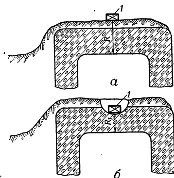
Рис. 227. Подрывание покрытий железобетонных фортификационных сооружений наружными зарядами:
