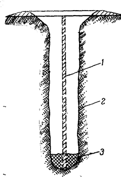
Рис. 114. Шахтный колодец, устраиваемый взрывом вертикально расположенного удлиненного заряда: 1 — положение заряда; 2 — контур колодца; 3 — обваливающийся после взрыва грунт
