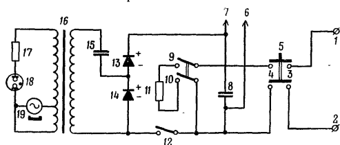
Рис. 39. Электрическая схема конденсаторной подрывной машинки КПМ-1 (приводная ручка вставлена):
