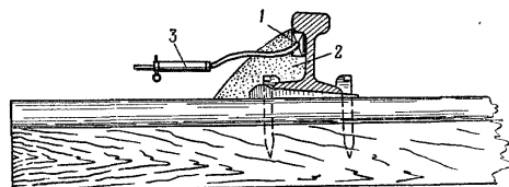
Рис. 198. Подрывание рельса: 1 — заряд; 2 — забивка; 3 — зажигательная трубка
