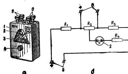
Рис. 52. Пульт для проверки подрывных машинок ПМ-1:
