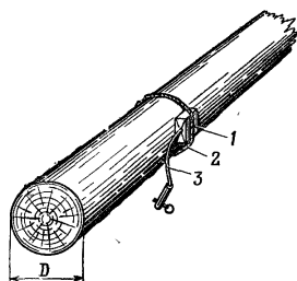
Рис. 66. Подрывание бревна сосредоточенным зарядом: 1 — заряд; 2 — проволока (шпагат); 3 — зажигательная трубка
