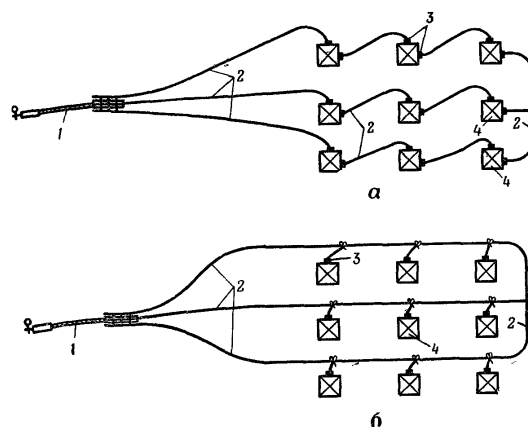
Рис. 32. Смешанные сети детонирующего шнура: а — для наружных зарядов; б — для внутренних зарядов; 1 — зажигательные трубки; 2 — отрезки детонирующего шнура; 3 — капсули-детонаторы; 4 — заряды ВВ
