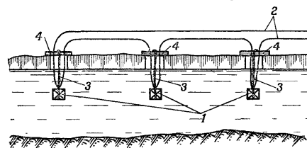
Рис. 243. Расположение группы зарядов для подрывания льда: 1 — заряды; 2 — провода; 3 — веревка; 4 — перекладины
