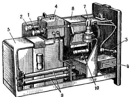
Рис. 41. Конденсаторная подрывная машинка КПМ-2 без корпуса:
