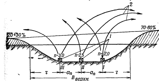
Рис. 105. Схема расположения зарядов для направленного выброса грунта (при одновременном взрывании): 1 — заряды; 2 — направление выброса основной массы грунта; I, II, III — номера рядов
