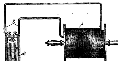
Рис. 35. Проверка целостности жилы сапёрного провода: 1 — провод на катушке; 2 — концы провода; 3 — малый омметр
