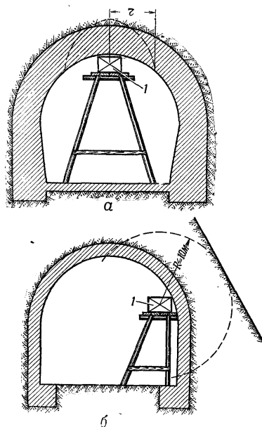
Рис. 179. Подрывание туннелей сосредоточенными зарядами, открыто располагаемыми у обделки: а — при прохождении туннеля в мягкой породе; б — то же, в твердой породе; I — заряды
