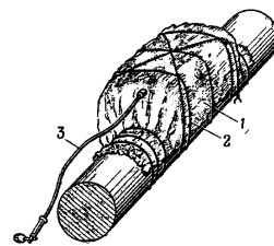
Рис. 83. Подрывание стального стержня зарядом из пластичного ВВ: 1 — заряд из пластита-4, обернутый тканью; 2 — шпагат; 3 — зажигательная трубка
