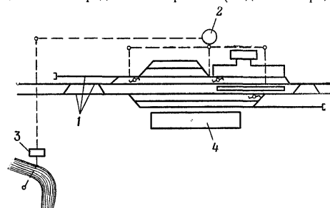
Рис. 211. Схема расположения объектов разрушения на железнодорожной станции: 1 — рельсовые пути; 2 — водонапорная башня; 3 — насосная станция; 4 — погрузочная площадка
