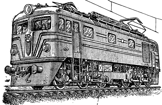
Рис. 203. Подрывание электровоза: I — заряд на моторно-осевых подшипниках
