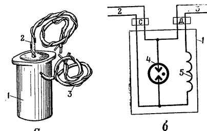
Рис. 64. Грозозащитный прибор ГЗУ: а — общий вид; б — электрическая схема; 1 — корпус; 2 — концы проводов с биркой С; 3 — концы проводов с биркой Д; 4 — неоновый разрядник; 5 — катушка индуктивности
