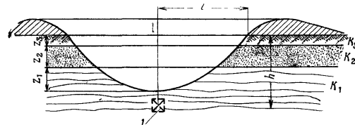
Рис. 97. Схема определения расчетного удельного расхода ВВ K_{расч} : 1 — положение заряда
