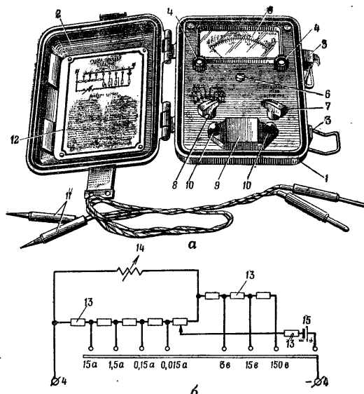
Рис. 53. Ампервольтметр (М-360):
