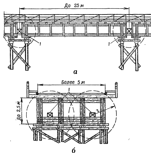
Рис. 132. Подрывание высоководного деревянного моста с дощато-гвоздевыми фермами: а — вид сбоку; б — поперечный разрез; 1 — заряды над опорами
