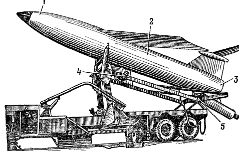
Рис. 238. Места расположения зарядов для подрывания пусковой установки с ракетой:
