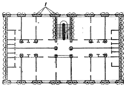
Рис. 123. Обрушение секции здания на месте подрыванием всех капитальных стен и колонн: I — заряды
