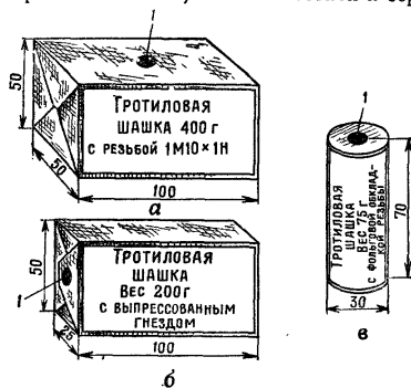
Рис. 1. Подрывные тротилевые шашки; а — большая; б — малая; в — буровая; 1 — запальное гнездо
