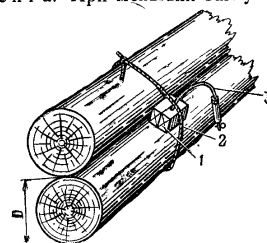
Рис. 73. Подрывание пакета из двух бревен:
