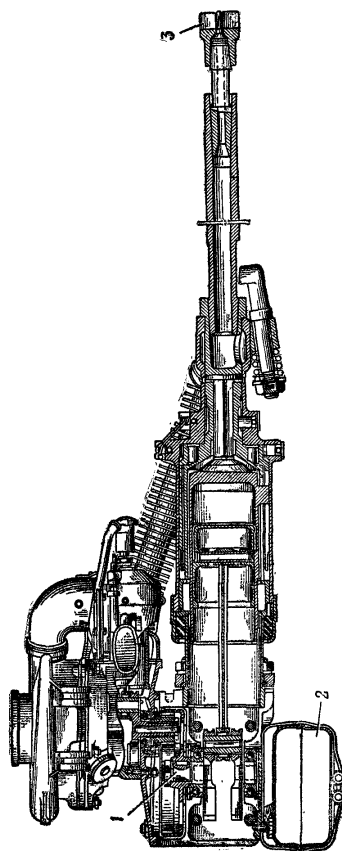
Рис. 274. Мотоперфоратор МПЛ: 1 — двигатель; 2 — бензобак; 3 — рабочий орган
