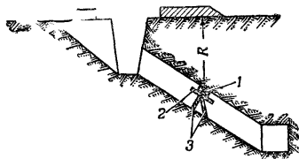
Рис. 230. Подрывание подземного убежища зарядом в наклонном входе: 1 — заряд; 2 — дощатая подкладка; 3 — подпорки
