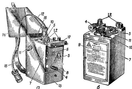
Рис. 37. Общий вид подрывной машинки КРМ-1: а — в футляре; б — без футляра; 1, 2 — линейные зажимы; 3 — пружинная заслонка; 4 — приводная ручка; 5 — окно неоновой лампы; 6 — кнопка взрыва; 7 — пластмассовый корпус; 8 — крышка (отъемная стенка) корпуса; 9 — металлическая пластинка с инструкцией; 10 — штепсельный разъем с контактами; 11 — заглушка штепсельного разъема; 12 — соединительный кабель с розетками; 13 — брезентовый футляр; 14 — крышка футляра; 15 — плечевой ремень; 16 — карманы для укладки пульта и соединительного кабеля; 17 — пульт
