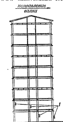
Рис. 129. Валка каркасного здания в сторону путем подрывания стоек каркаса в разных уровнях: I — заряды
