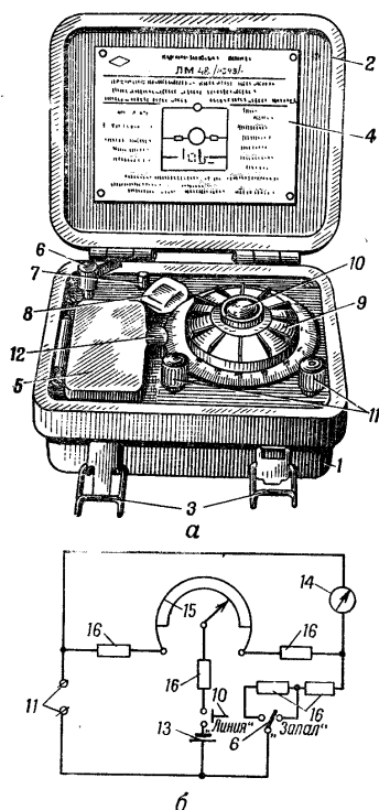
Рис. 48. Линейный мост ЛМ-48 (Р-343): а — общий вид с открытой крышкой; б — электрическая схема; 1 — корпус; 2 — крышка; 3 — замки; 4 — щиток с инструкцией; 5 — крышка камеры источника тока; 6 — ручка переключателя пределов измерения; 7 — корректор; 8 — окно нулевого прибора; 9 — лимб со шкалами делений; 10 — кнопка включения источника тока; 11 — зажимы для подключения измеряемых сопротивлений; 12 — винт, запирающий крышку камеры источника тока; 13 — источник тока; 14 — нулевой прибор (гальванометр); 15 — реохорд; 16 — сопротивления
