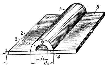
Рис. 16. Удлиненныйкумулятивный заряд из пластита-4: 1 — заряд; 2 — запальное гнездо; 3 —кумулятивная полость; 4 —металлическая обкладка; 5 —перебиваемый лист
