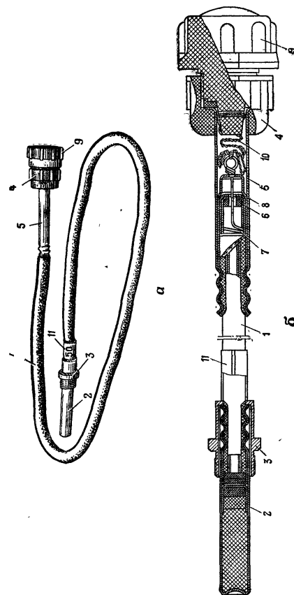
Рис. 24. Зажигательная трубка с терочным воспламенителем: а — общий вид; б — разрез. 1 — огнепроводный шнур; 2 — капсюль-детонатор № 8-А; 3 — ниппель; 4 — корпус; 5 — трубка; 6 — терочный капсюль-вспламенитель; 7 — запорный винт; 8 — винт; 9 — алюминиевая муфта; 10 — винт; 11 — указывающая время замедления в секундах
