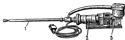
Рис. 275. Электроперфоратор С-408Б: 1 — рабочий орган; 2 — стальной ствол; 3 — алюминиевый корпус
