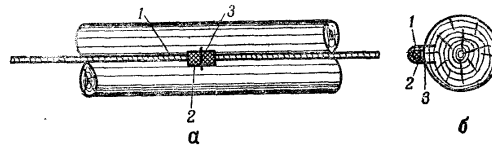
Рис. 137. Крепление проводов и детонирующего шнура к элементам деревянных мостов: а — вид сбоку; б — поперечный разрез; 1 — провод (детонирующий шнур); 2 — защитная накладка; 3 — проводочная скоба
