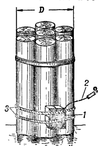
Рис. 71. Подрывание сосредоточенного куста свай контактным зарядом:
