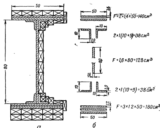
Рис. 80. Схема расчета и составления фигурного заряда для подрывания двутавровой стальной балки: а — поперечный разрез балки с расположением шашек ВВ (крепление не показано); б — схема вычисления площадей поперечного сечения элементов балки
