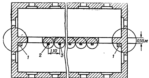
Рис. 122. Повреждение здания подрыванием внутренней капитальной стены: 1, 2, 3 — заряды
