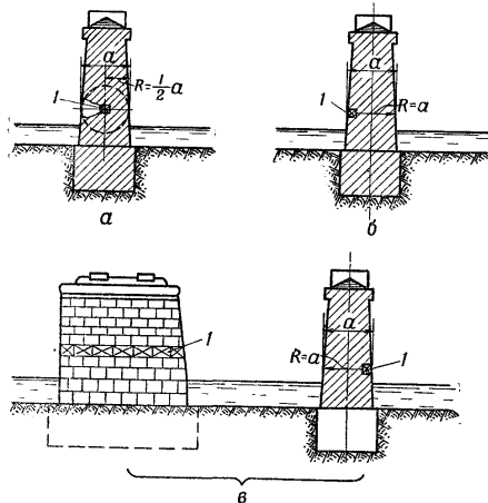
Рис. 150. Подрывание промежуточных мостовых опор (быков) по всей ширине в одном уровне: а — сосредоточенными зарядами в нишах; б — сосредоточенными зарядами в борозде; в — удлиненным зарядом в борозде; 1 — заряды
