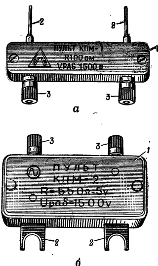
Рис. 51. Пульты для проверки подрывных машинок: а — КИМ-1; б — КИМ-2; 1 — корпус; 2 — контакты для подключения пультов к машинкам; 3 — клеммы для подключения электродетонаторов
