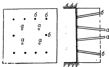
Рис. 110. Схема расположения шпуров при проходке галерей: a — врубные шпуры; b — отбойные шпуры
